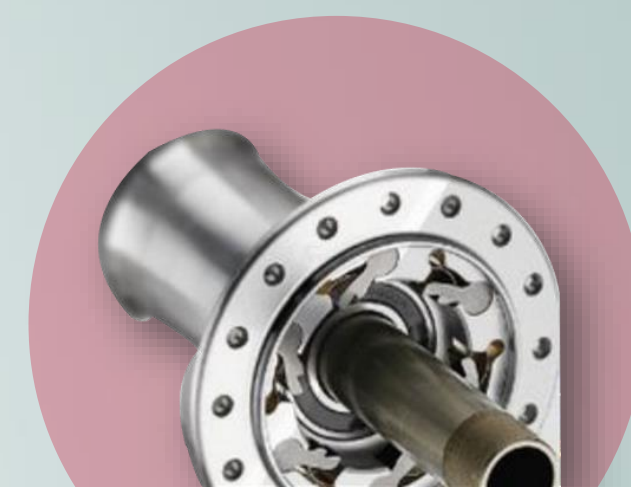
自行車發電 (輪鼓馬達)
